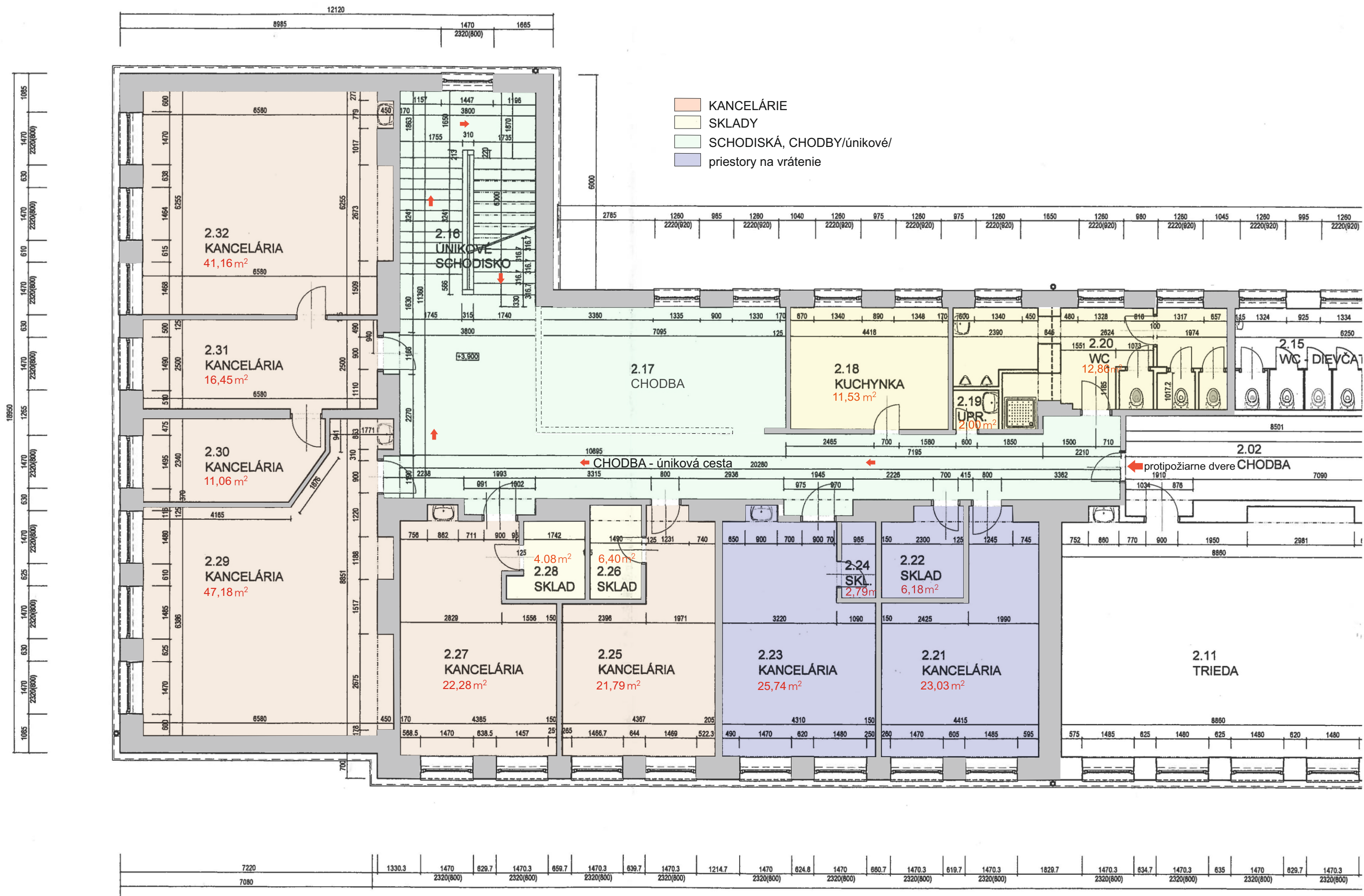
Pôdorys 1.NP
